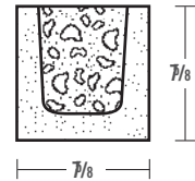
.22 cu.ft. concrete per lin. ft.
