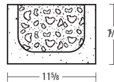
.37 cu.ft. concrete per lin. ft.
