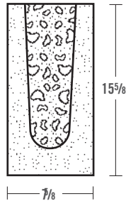
.46 cu.ft. concrete per lin. ft.
